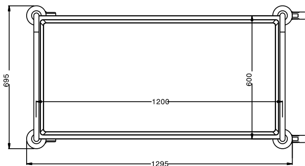
Boven aanzicht
